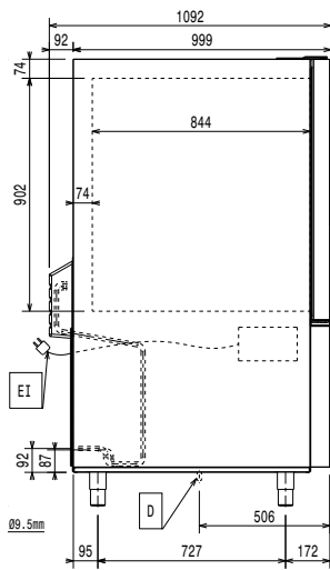
Oldalnézet
