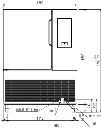
Előlnézet
